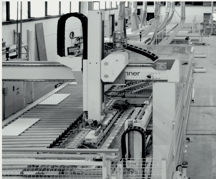
Macchina squadrabordatrice Squaring edgebanding machine
