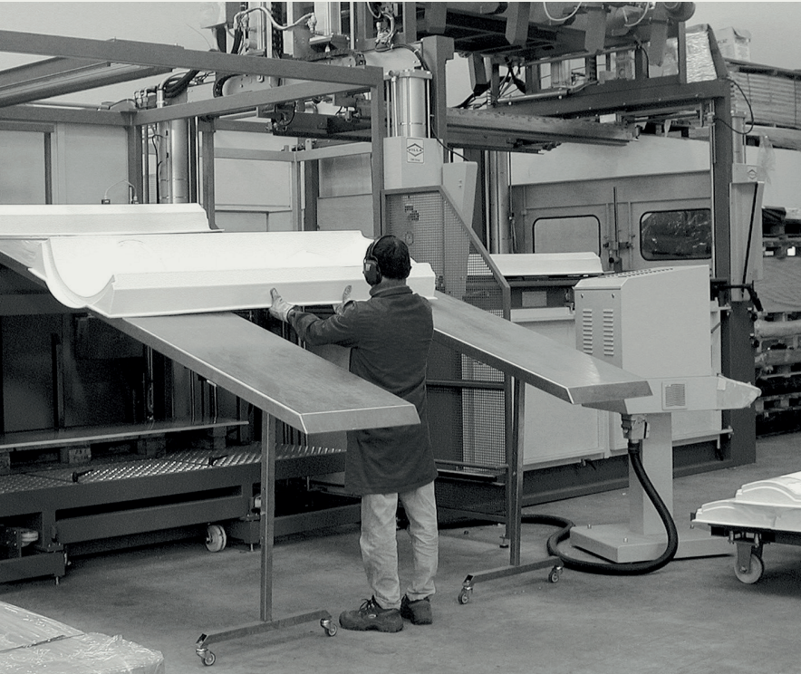
Impianto di termoformatura per materiali acrilici Thermoforming plant for acrylic materials
