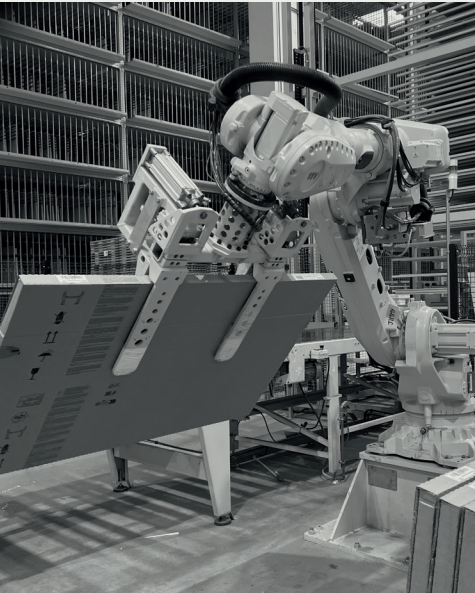
Nuovo impianto di imballaggio New packaging plant
