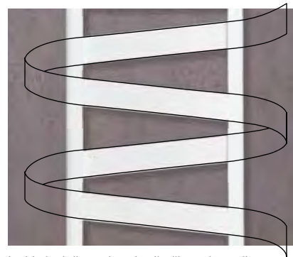
I tubi piatti disposti su due livelli avvolgono il radiatore da bagno Zehnder Ribbon come un nastro d'acciaio.
